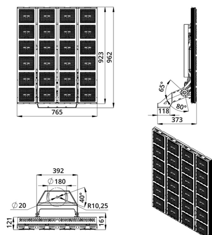
Габаритный чертеж
