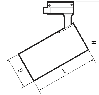
Рис. 1 Прожектор PTR 07
