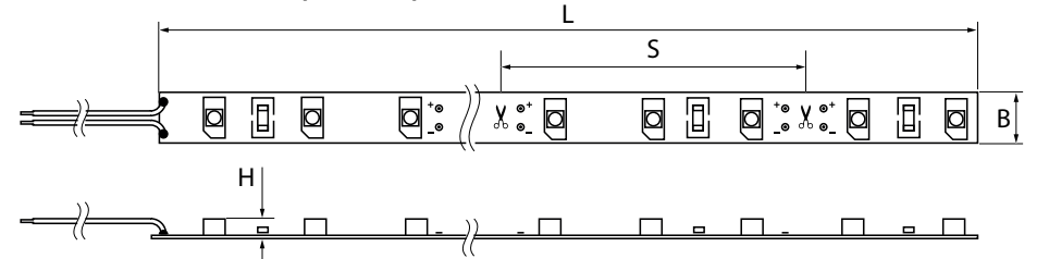
Рис. 1 Лента светодиодная
